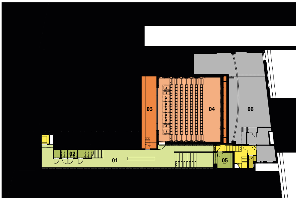
Sous-sol 01: foyer 02: sanitaires 03: projection/régie/prép. 04: petite salle 05: bar/caisse 06: locaux techniques
